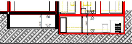
SNITT D - D
