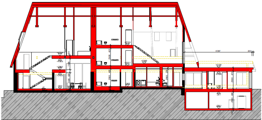
SNITT A - A
