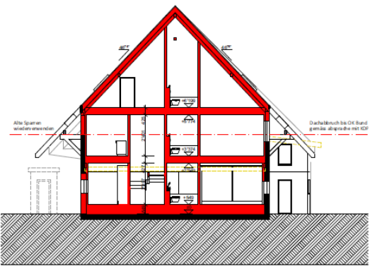
SNITT B - B
